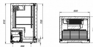
Стал бальный TM101/2-дверная дверь без стол-цы
