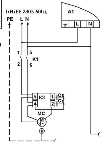
Рис.2 (однофазное питание) остальное см. рис.1
