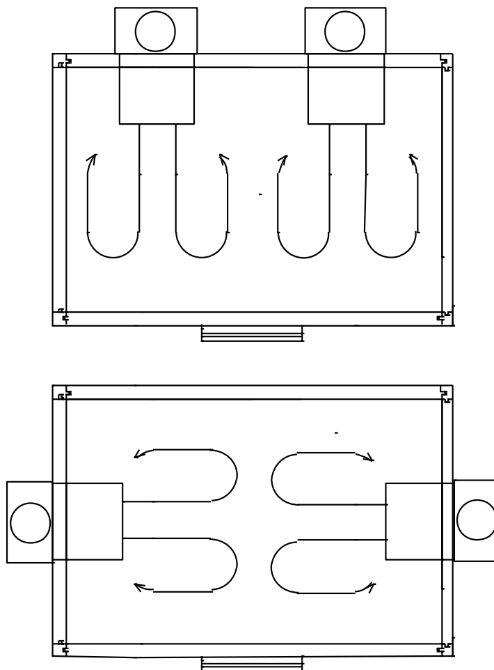
Рис.17 Варианты установки двух однотипных машин в одну камеру
