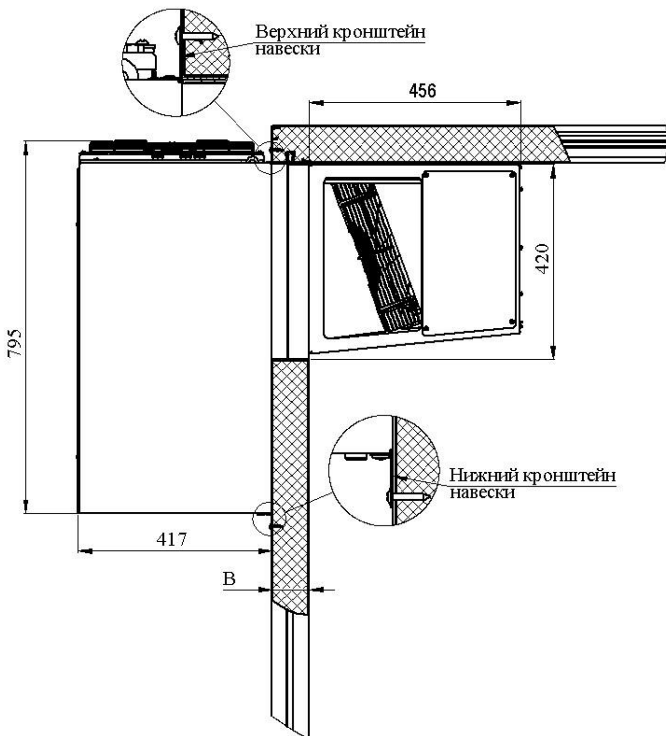
Рис.14 Схема установки моноблока 330 серии.
