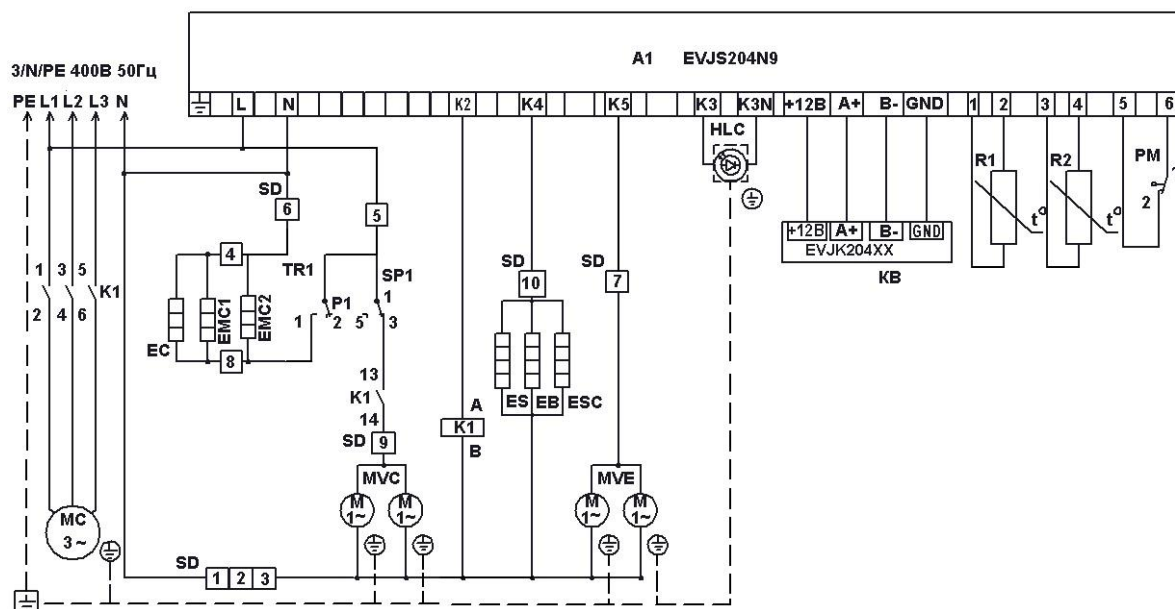
Рис.1. (трехфазное питание)
