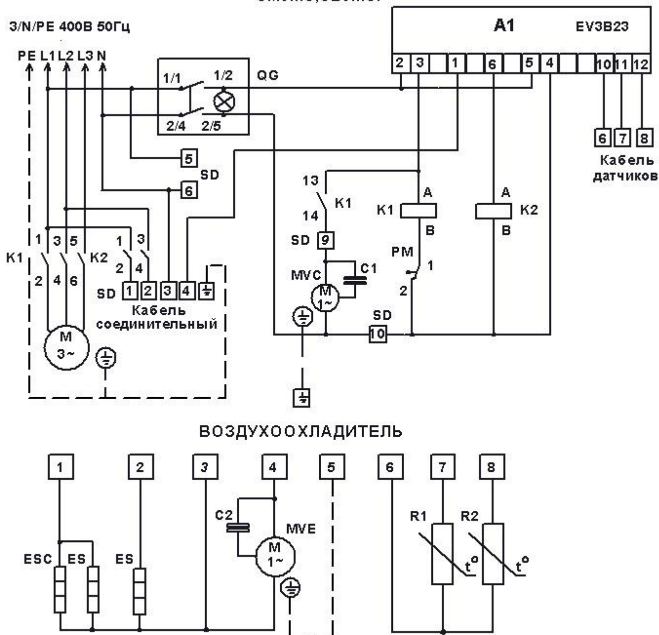
Рис.6 Схема электрическая принципиальная сплит-систем SM3...S, SB3...S.
