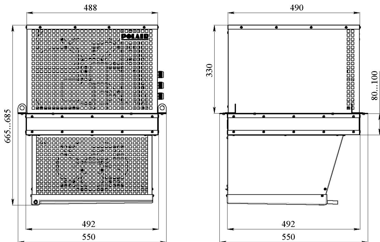
Рис.2 Габаритные размеры потолочных моноблока 1-го типоразмера
